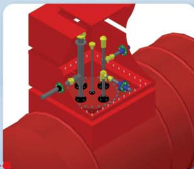
Installazione di serbatoi da 50mc Installation of 50m3 PetrolTank
